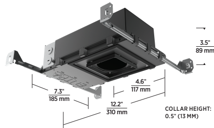
IC AIRTIGHT/ CHICAGO PLENUM
